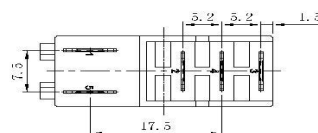
安装尺寸 (底视)
