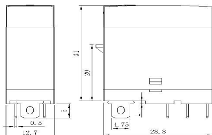
NNC69KTL-1Z 外形尺寸
